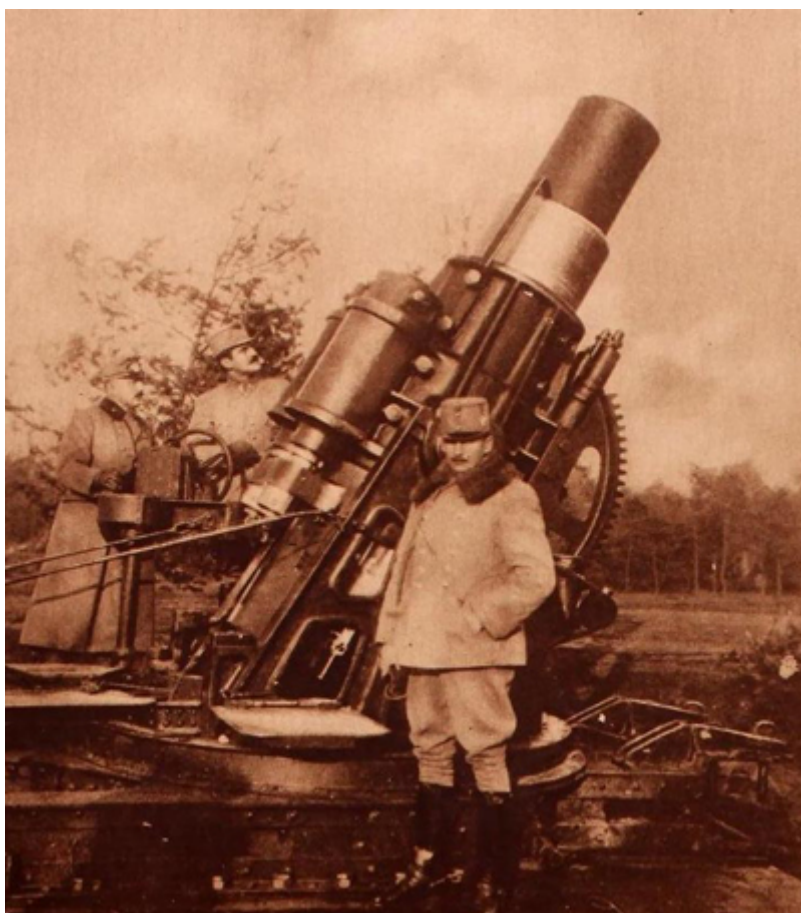
Houfnice ráže 38 cm Škoda - dobová fotografie, zdroj: Sbírka Gantschacher
